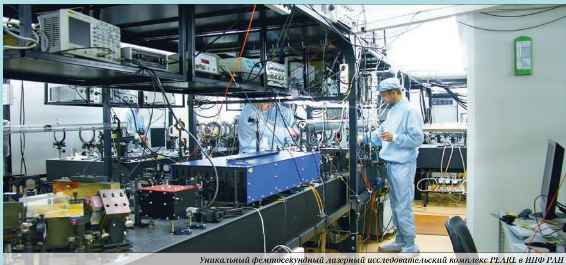
Уникальный фемтосекундный лазерный исследовательский комплекс PEARL в ИПФ РАН
